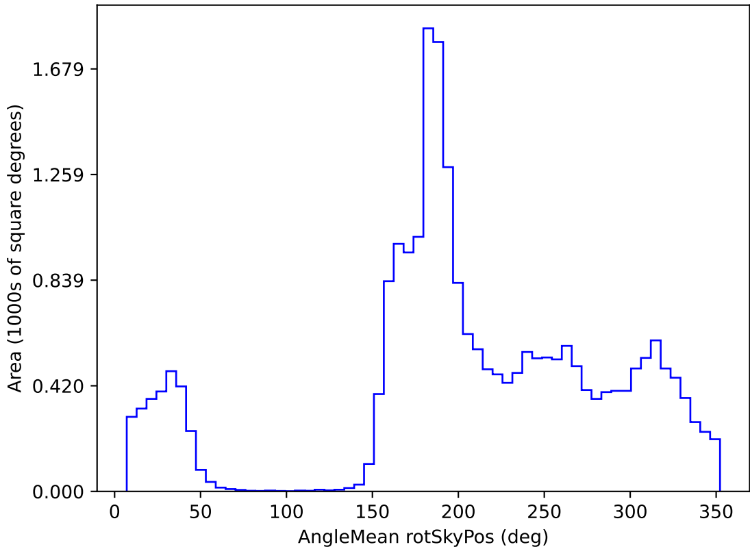
weather_cloudso18v3.4_10yrs All sky y band: AngleMean rotSkyPos
