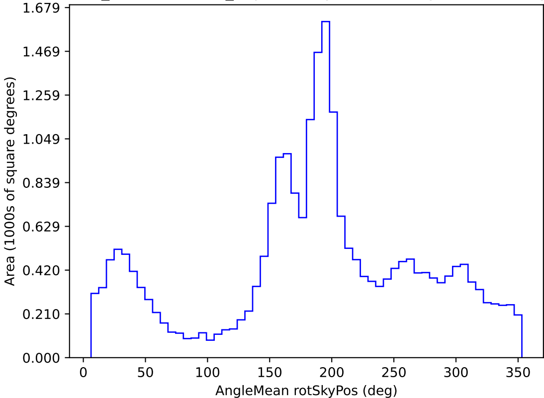
weather_cloudso18v3.4_10yrs All sky u band: AngleMean rotSkyPos
