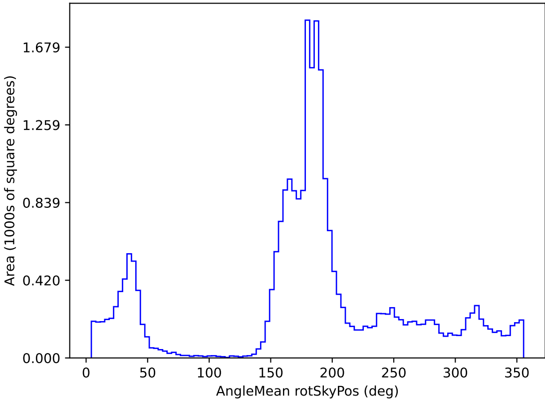
weather_cloudso18v3.4_10yrs All sky r band: AngleMean rotSkyPos
