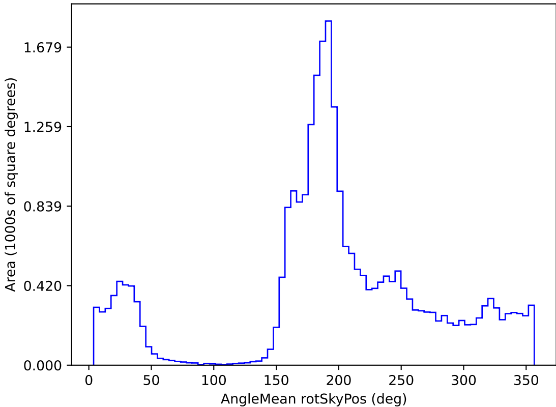
weather_cloudso18v3.4_10yrs All sky i band: AngleMean rotSkyPos
