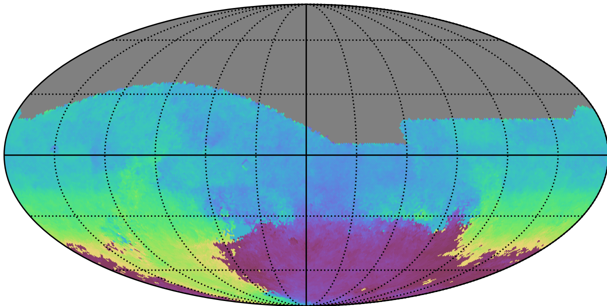
weather_cloudso18v3.4_10yrs All sky g band: AngleMean rotSkyPos
