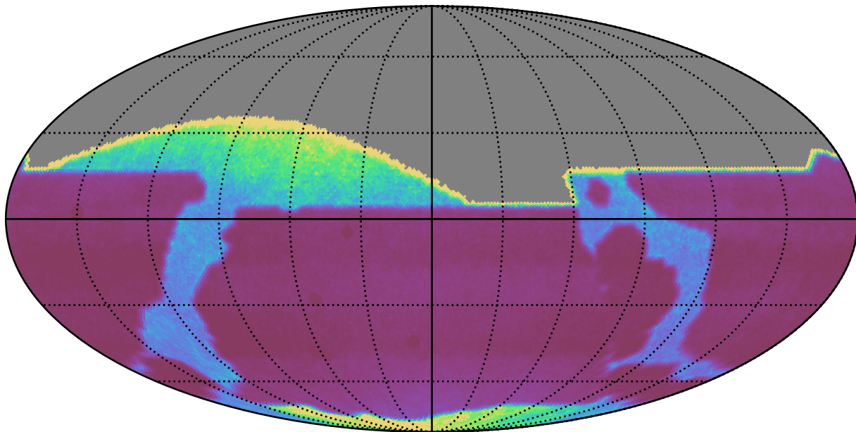
weather_cloudso18v3.4_10yrs : properMotion
