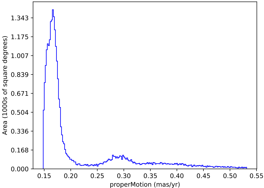
weather_cloudso18v3.4_10yrs : properMotion
