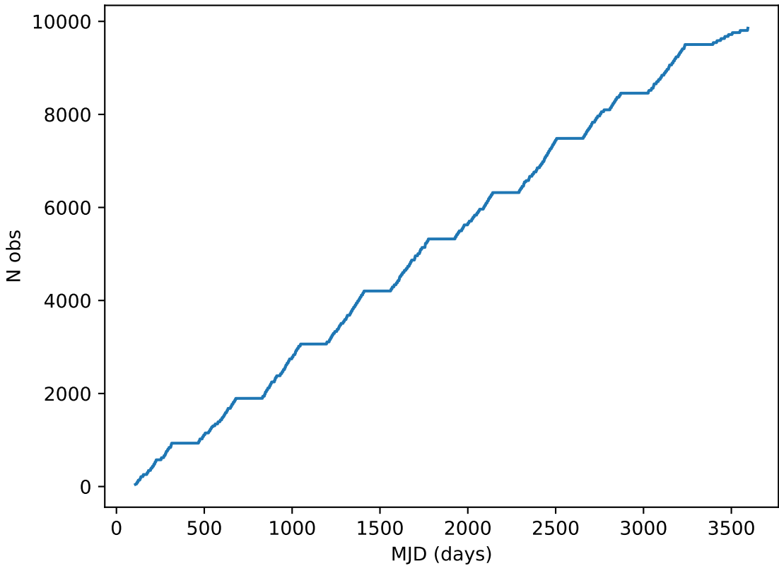
weather_cloudso18v3.4_10yrs note like DD:EDFS_b%: Cumulative
