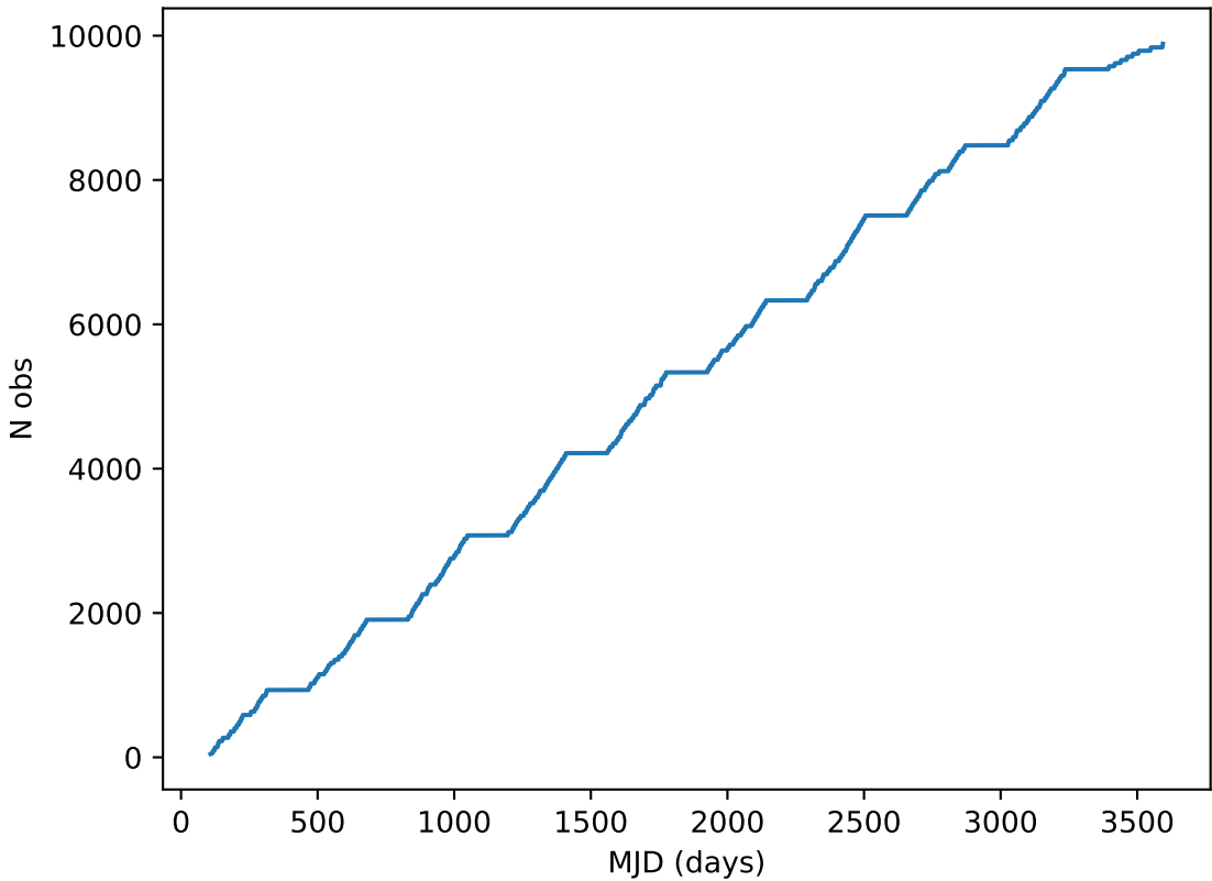
weather_cloudso18v3.4_10yrs note like DD:EDFS_a%: Cumulative
