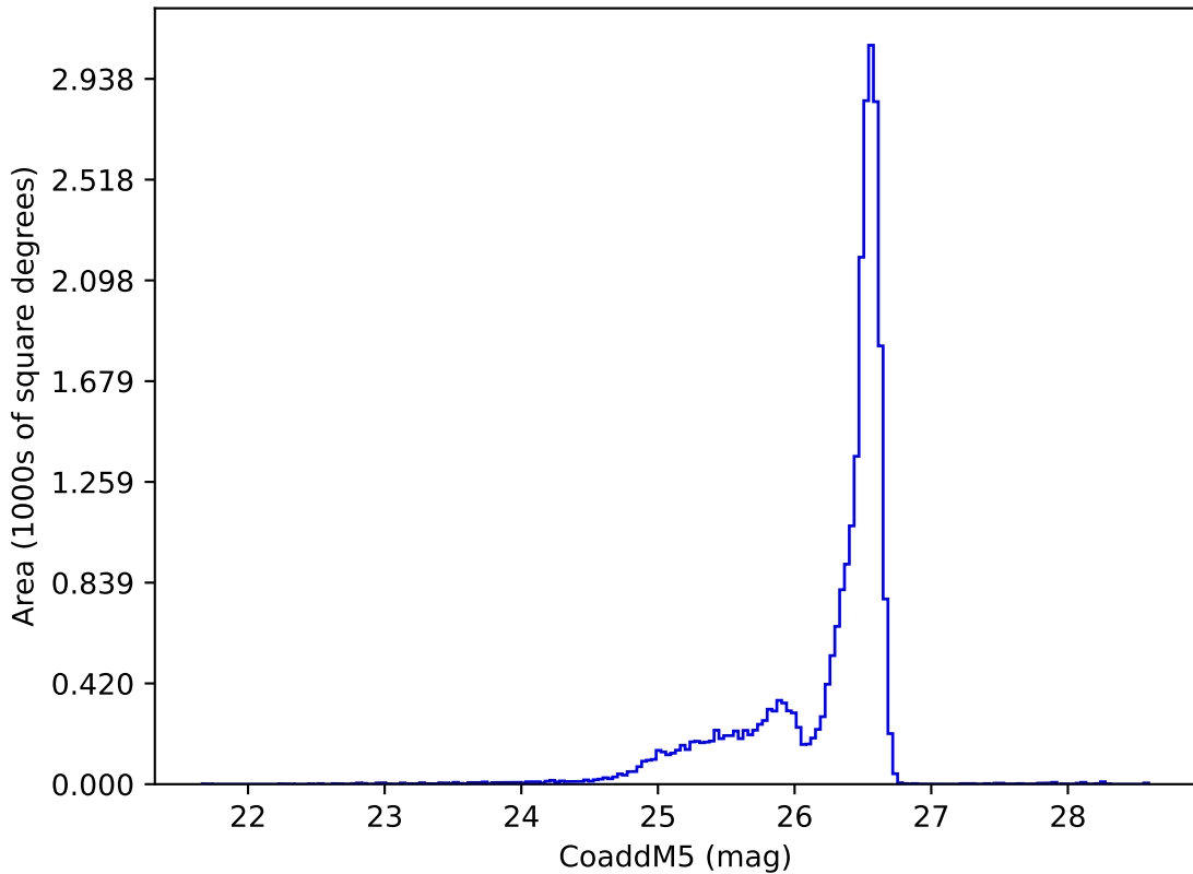
weather_cloudso18v3.4_10yrs i: CoaddM5
