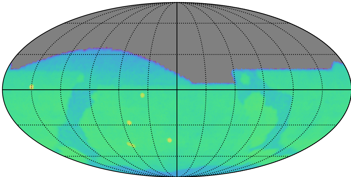
weather_cloudso18v3.4_10yrs g: CoaddM5
