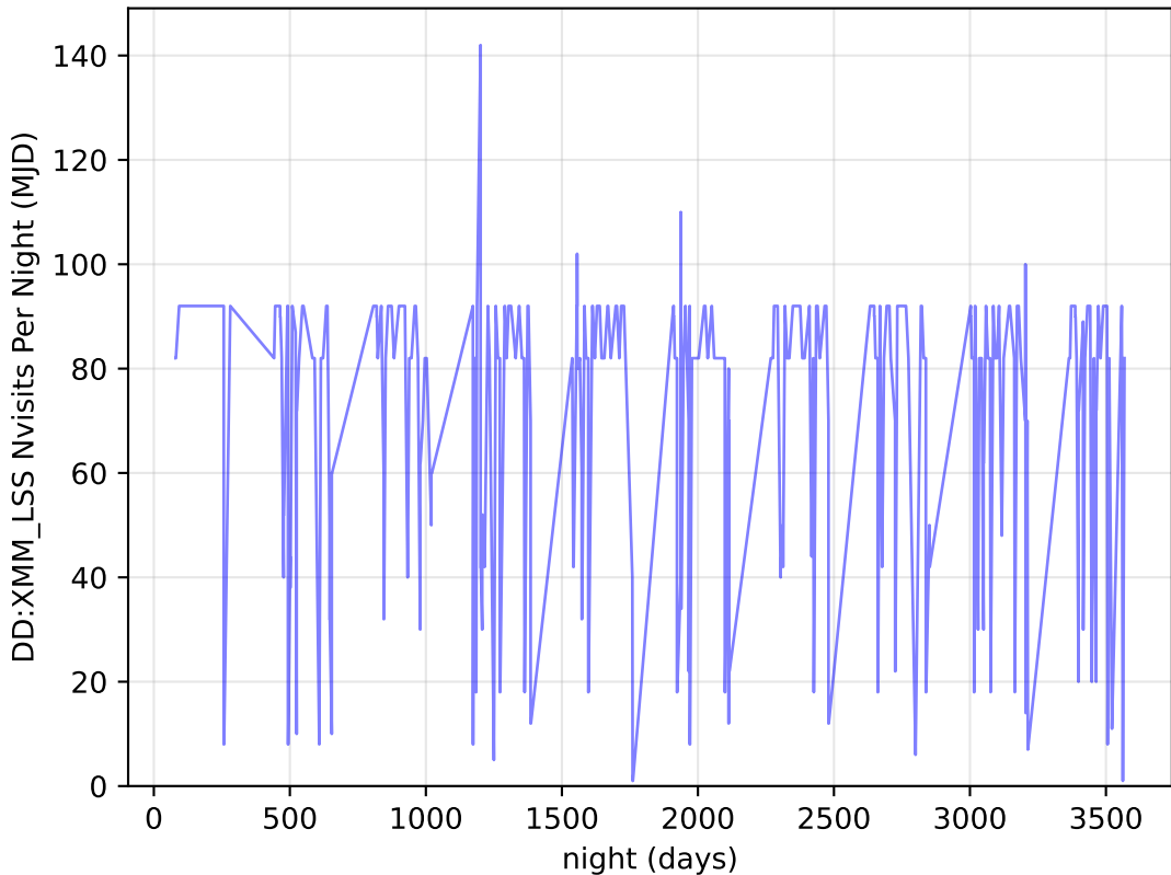
weather_cloudso18v3.4_10yrs all bands: DD:XMM_LSS Nvisits Per Night
