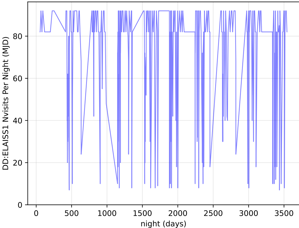
weather_cloudso18v3.4_10yrs all bands: DD:ELAISS1 Nvisits Per Night
