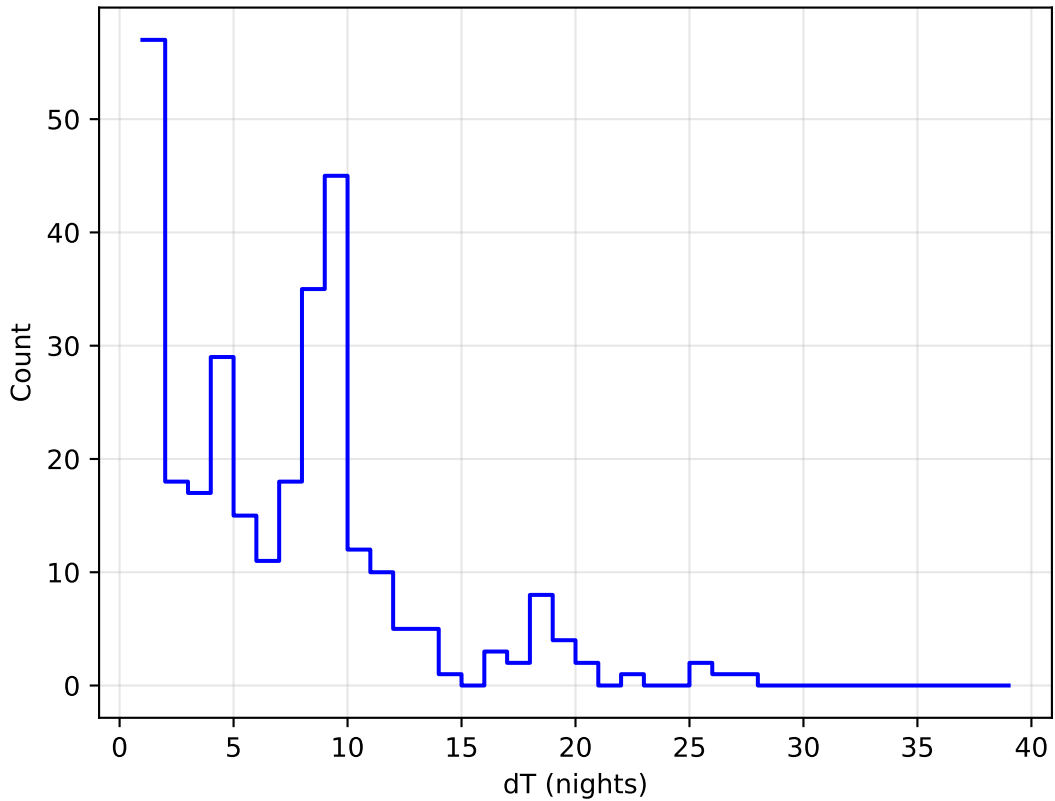
weather_cloudso18v3.4_10yrs all bands: DD:ELAISS1 Delta Nights Histogram
