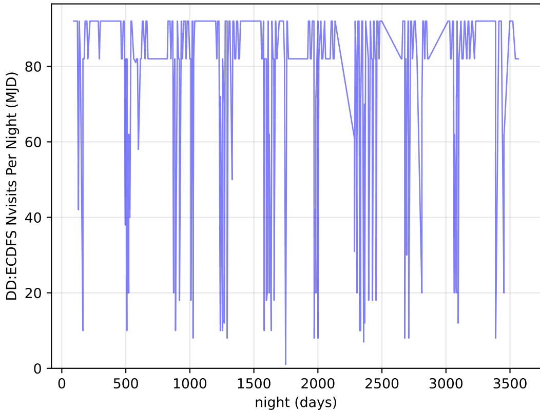
weather_cloudso18v3.4_10yrs all bands: DD:ECDFS Nvisits Per Night
