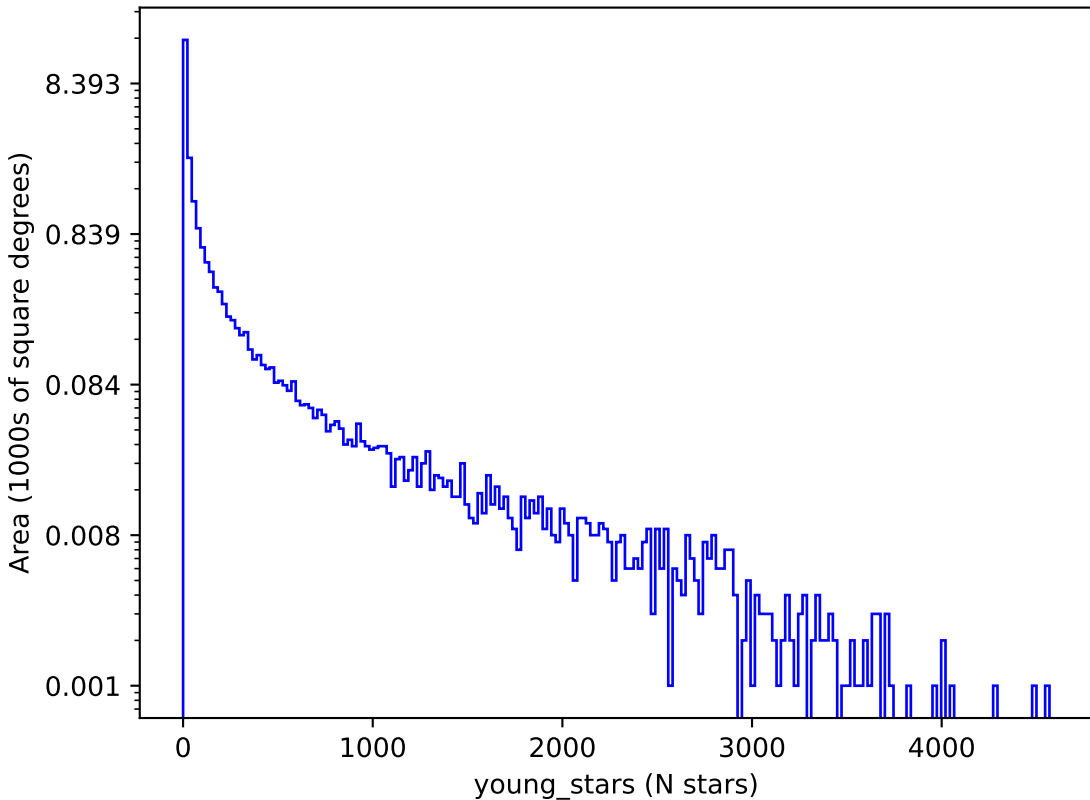
weather_cloudso16v3.4_10yrs : young_stars
