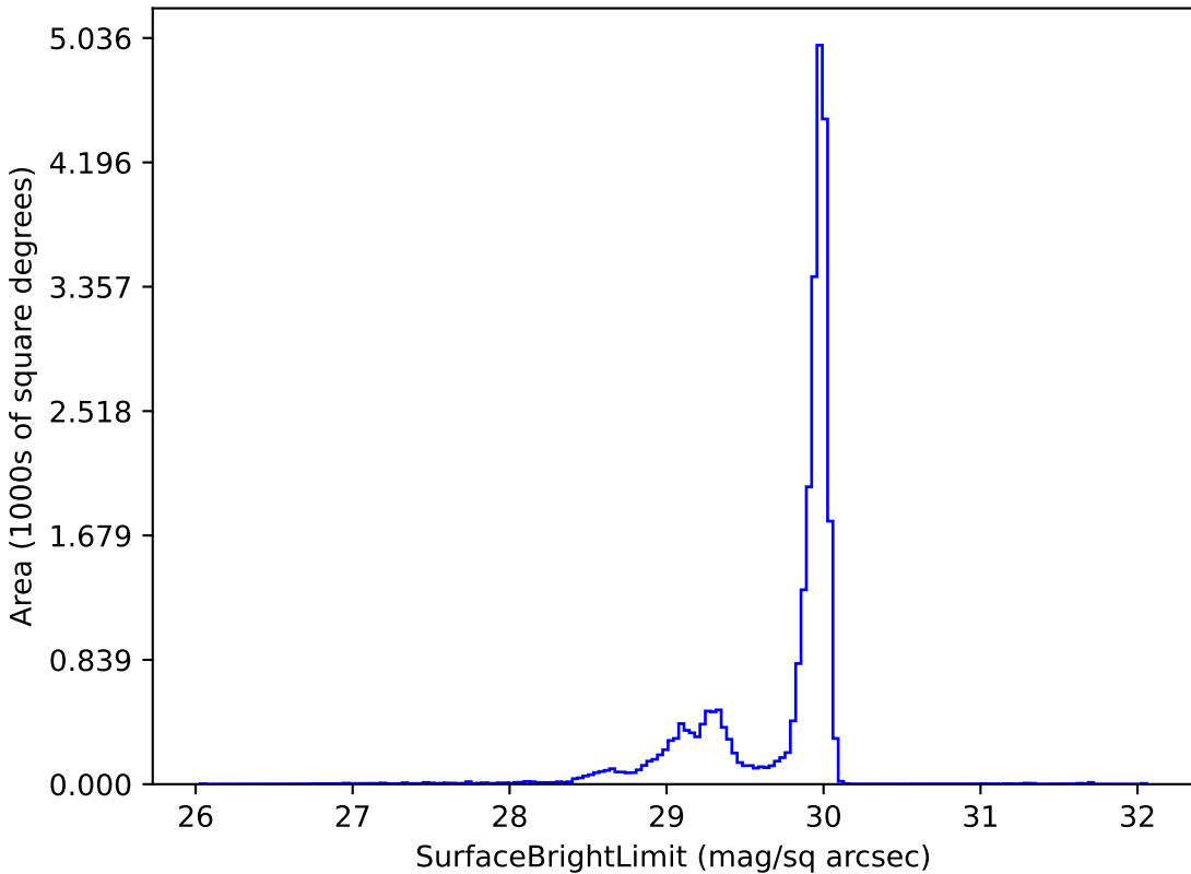
weather_cloudso16v3.4_10yrs i: SurfaceBrightLimit
