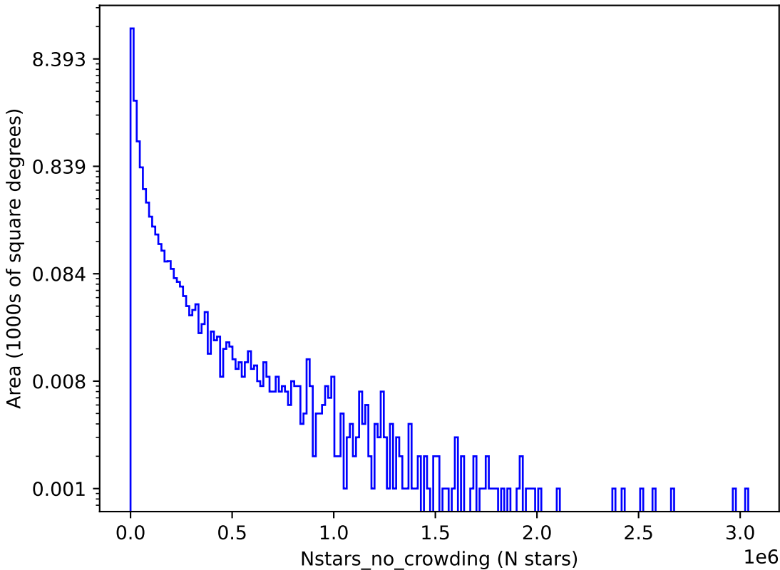
weather_cloudso16v3.4_10yrs u: Nstars_no_crowding
