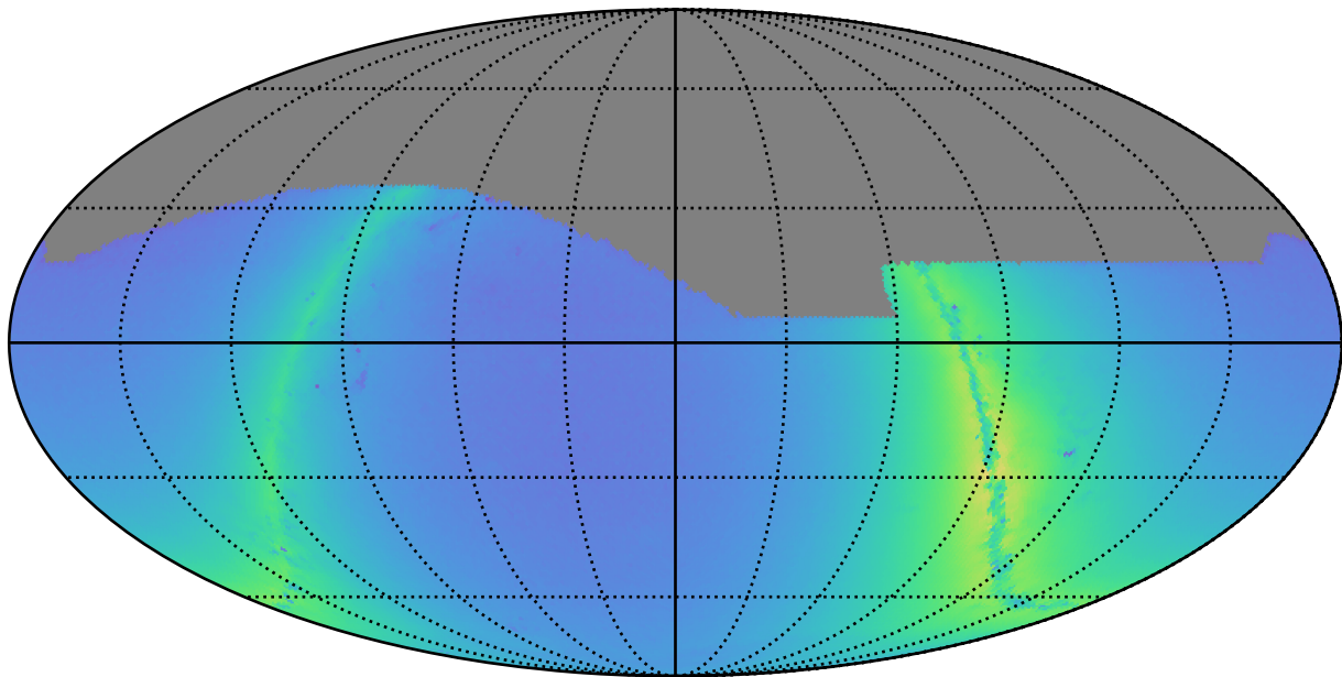
weather_cloudso16v3.4_10yrs r: Nstars_no_crowding
