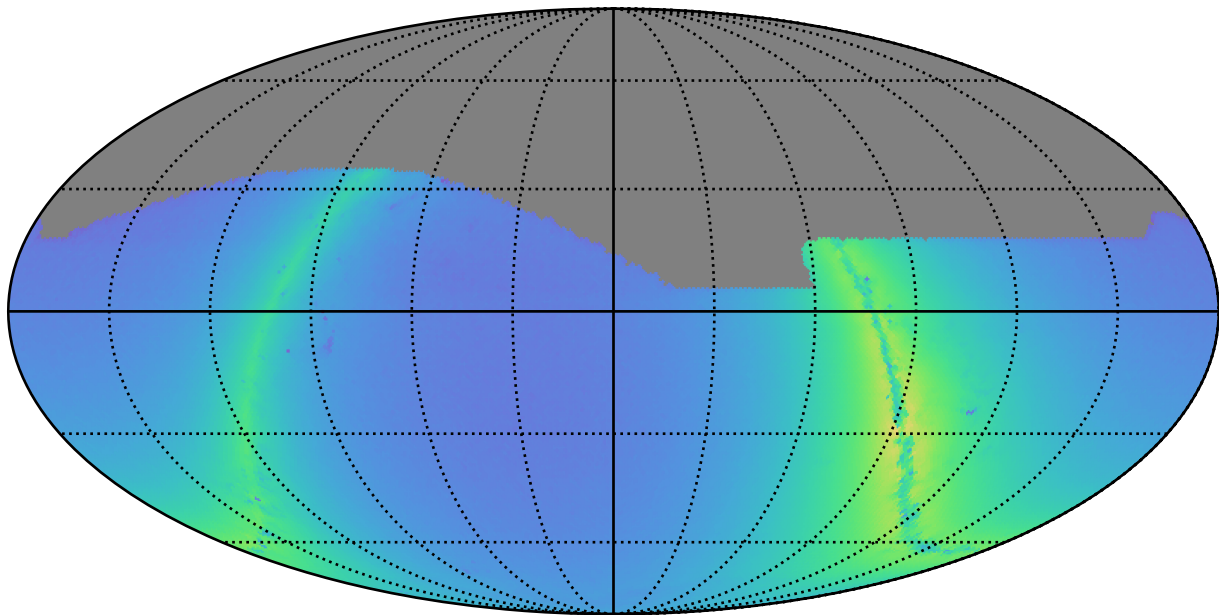
weather_cloudso16v3.4_10yrs i: Nstars_no_crowding
