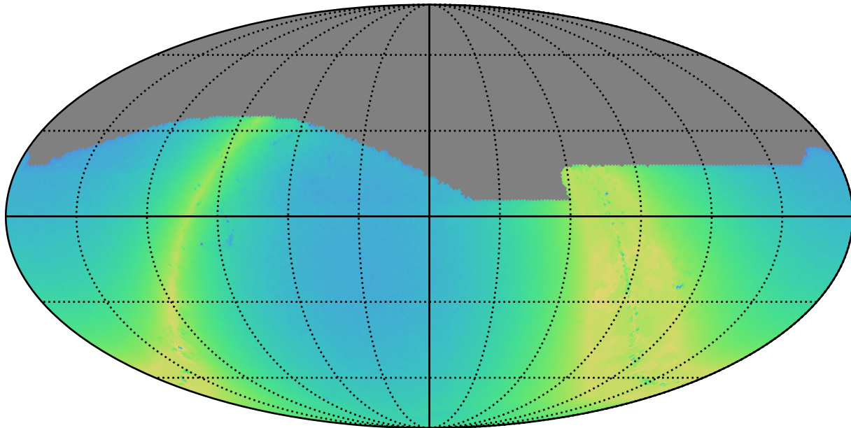
weather_cloudso16v3.4_10yrs i: N stars to Precision 0.20
