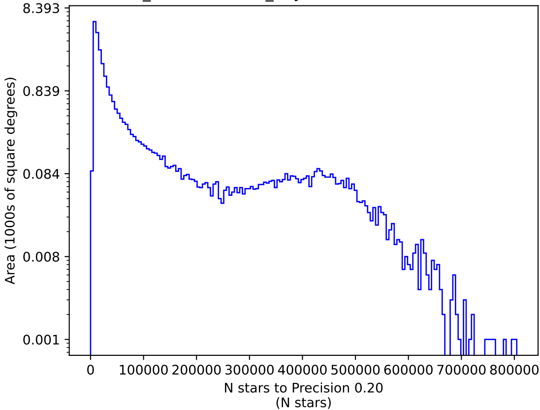
weather_cloudso16v3.4_10yrs i: N stars to Precision 0.20
