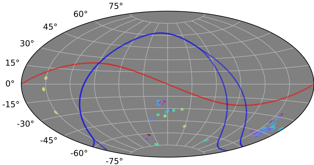
weather_cloudso16v3.4_10yrs gi: LVDwarfs
