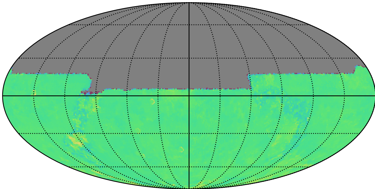
weather_cloudso16v3.4_10yrs u: Kuiper rotTelPos
