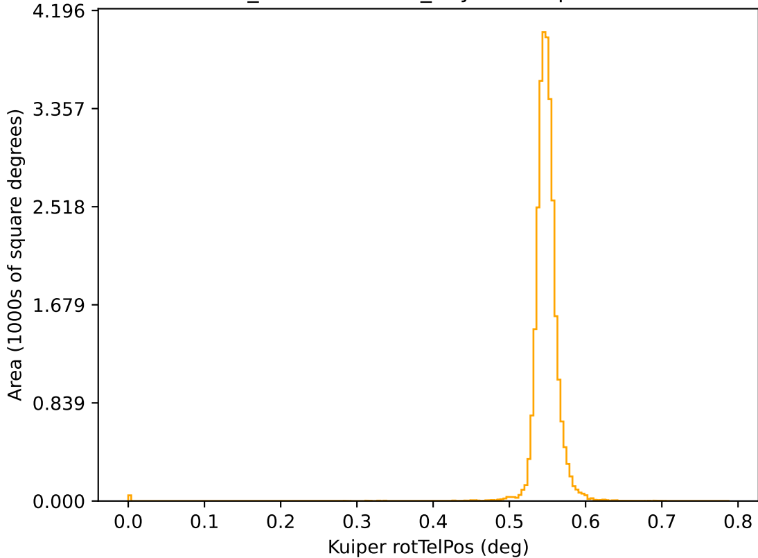
weather_cloudso16v3.4_10yrs r: Kuiper rotTelPos
