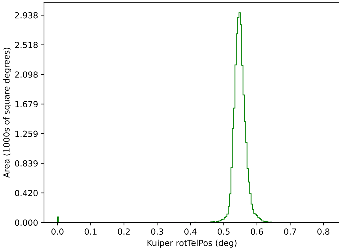
weather_cloudso16v3.4_10yrs g: Kuiper rotTelPos
