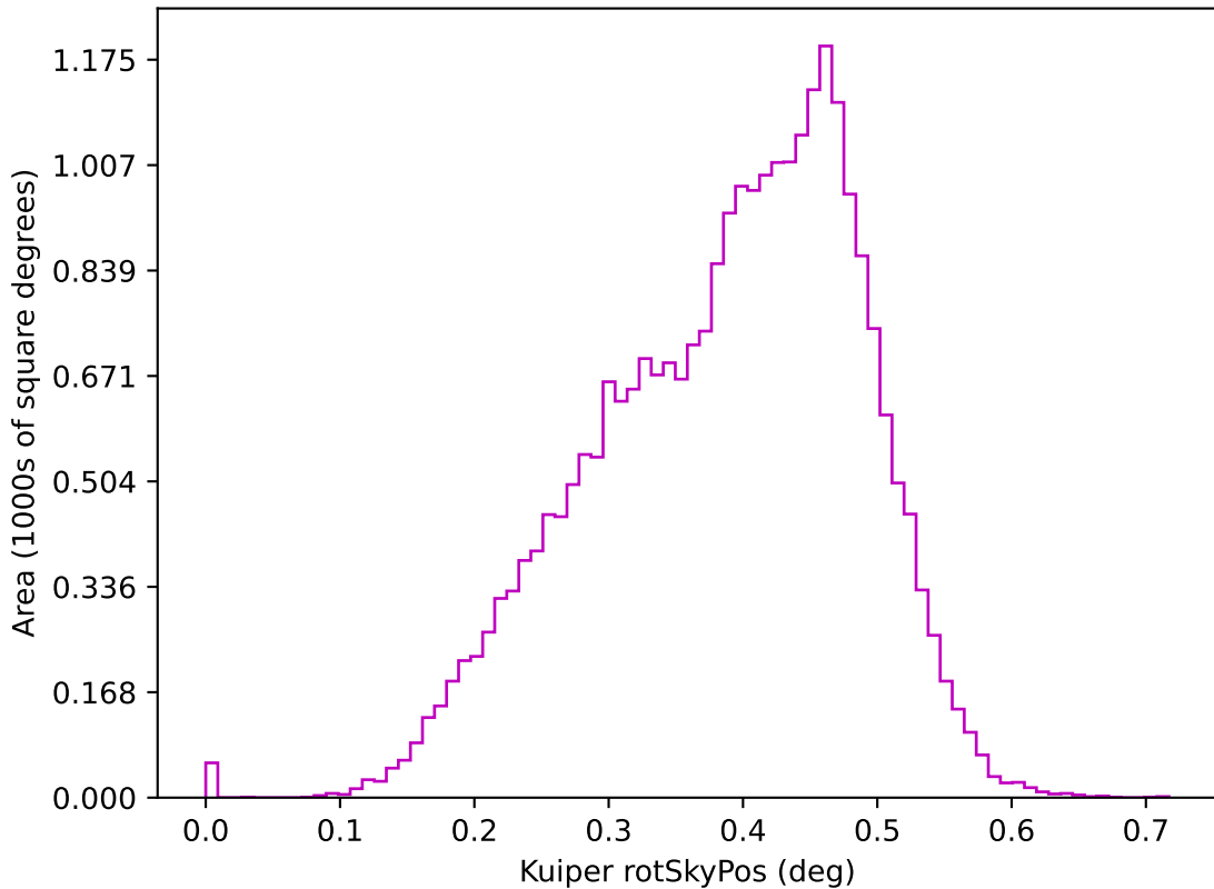
weather_cloudso16v3.4_10yrs z: Kuiper rotSkyPos
