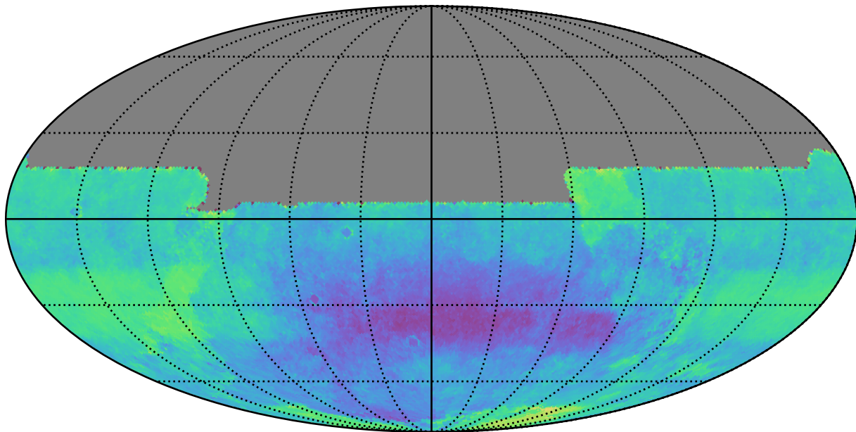
weather_cloudso16v3.4_10yrs y: Kuiper rotSkyPos
