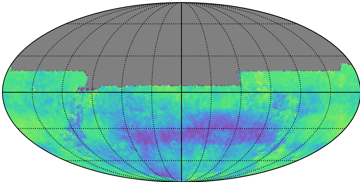
weather_cloudso16v3.4_10yrs u: Kuiper rotSkyPos
