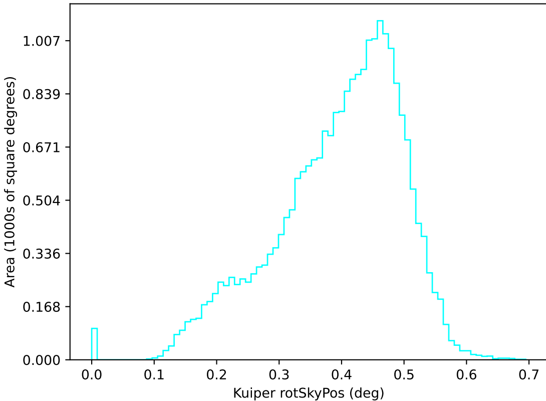
weather_cloudso16v3.4_10yrs u: Kuiper rotSkyPos
