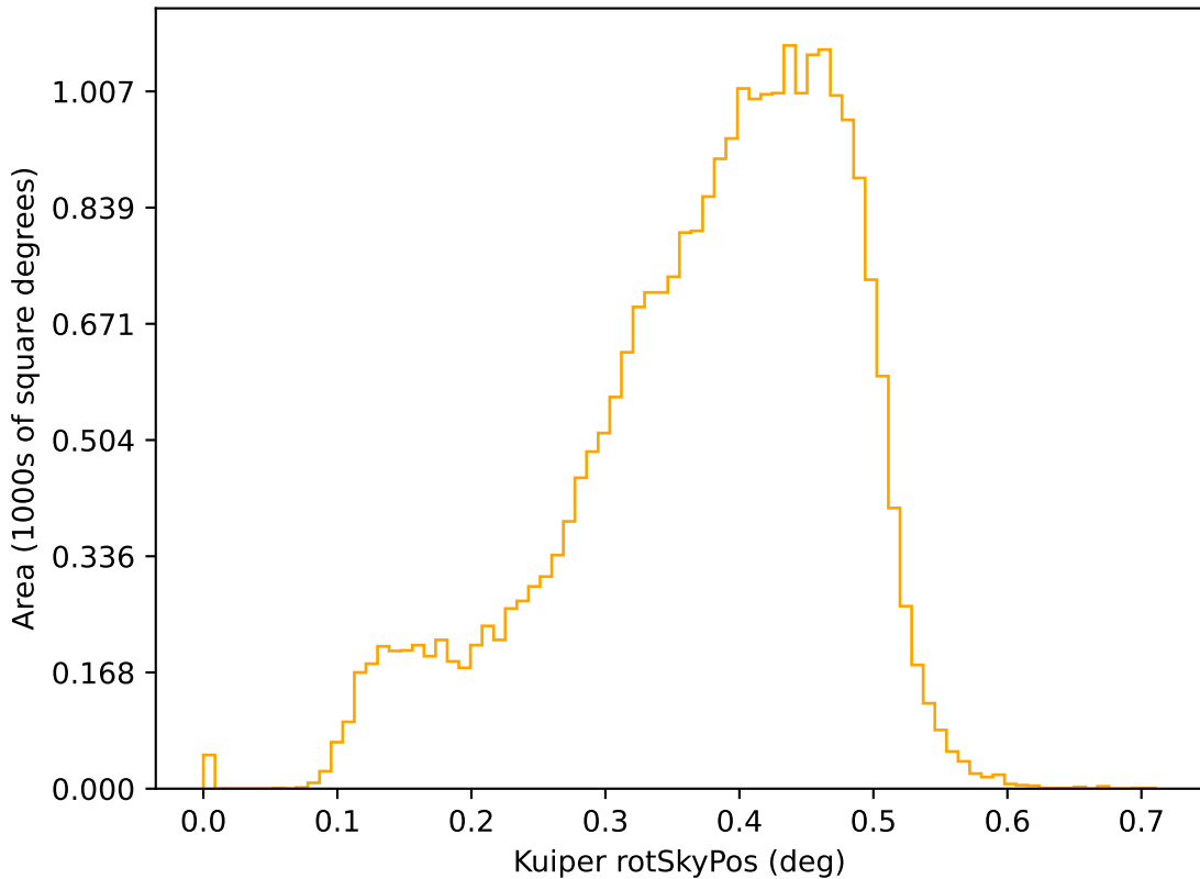
weather_cloudso16v3.4_10yrs r: Kuiper rotSkyPos
