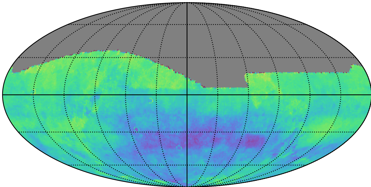
weather_cloudso16v3.4_10yrs i: Kuiper rotSkyPos
