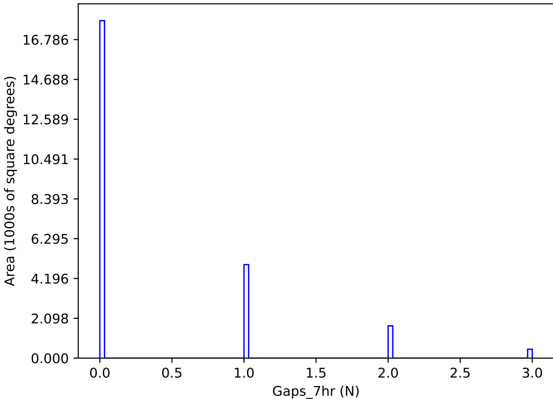
weather_cloudso16v3.4_10yrs y band: Gaps_7hr
