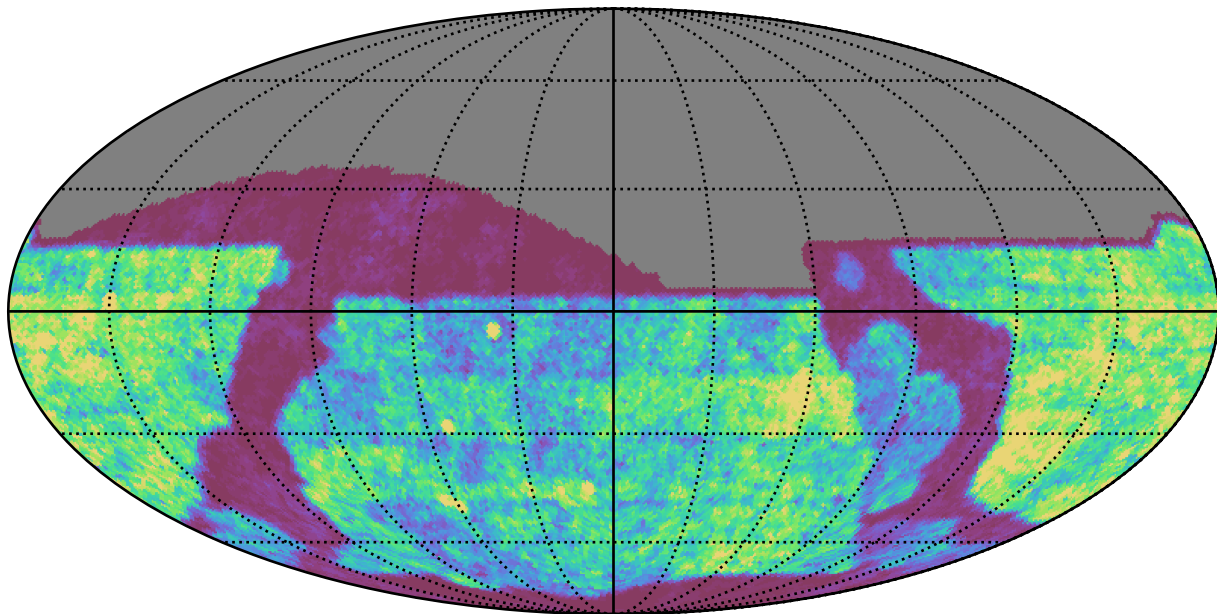
weather_cloudso16v3.4_10yrs z band: Gaps_24hr
