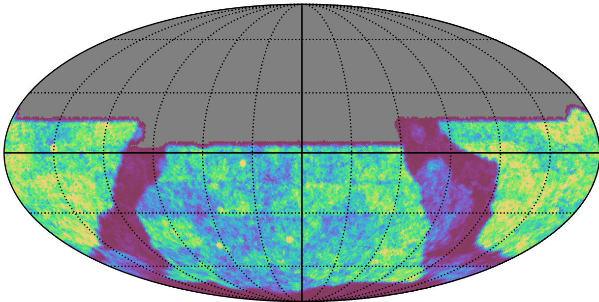
weather_cloudso16v3.4_10yrs y band: Gaps_24hr
