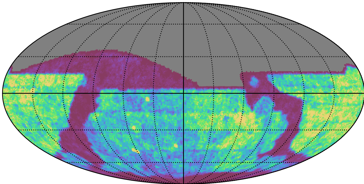
weather_cloudso16v3.4_10yrs i band: Gaps_24hr
