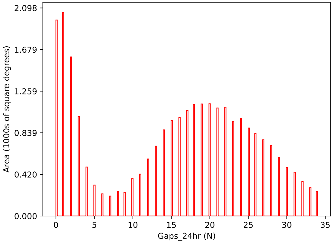
weather_cloudso16v3.4_10yrs i band: Gaps_24hr
