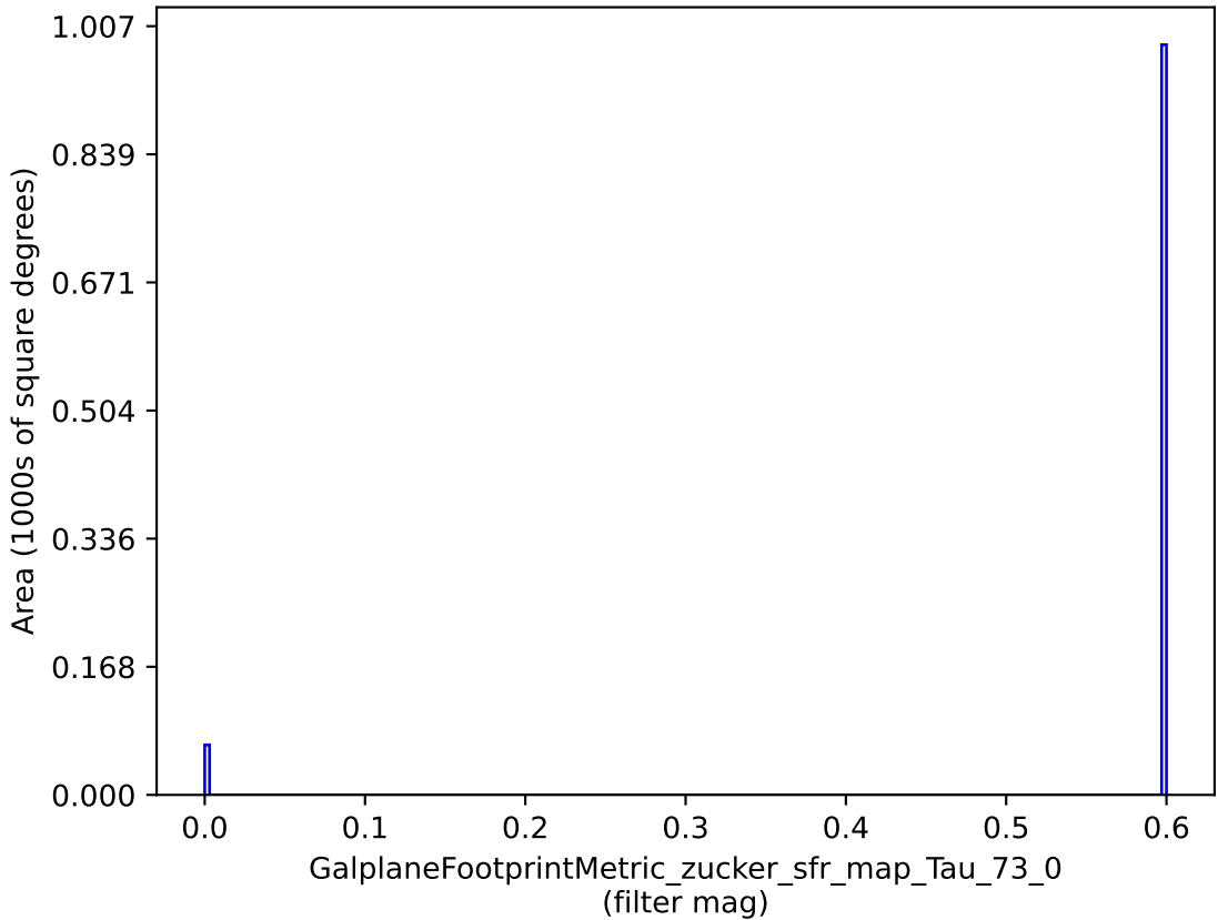
weather_cloudso16v3.4_10yrs : GalplaneFootprintMetric_zucker_sfr_map_Tau_73_0
