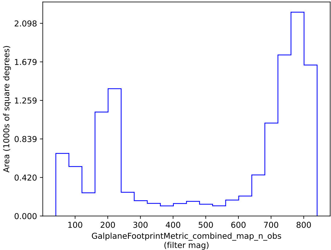
weather_cloudso16v3.4_10yrs : GalplaneFootprintMetric_combined_map_n_obs
