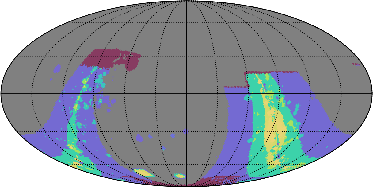
weather_cloudso16v3.4_10yrs : GalplaneFootprintMetric_combined_map_Tau_46_5
