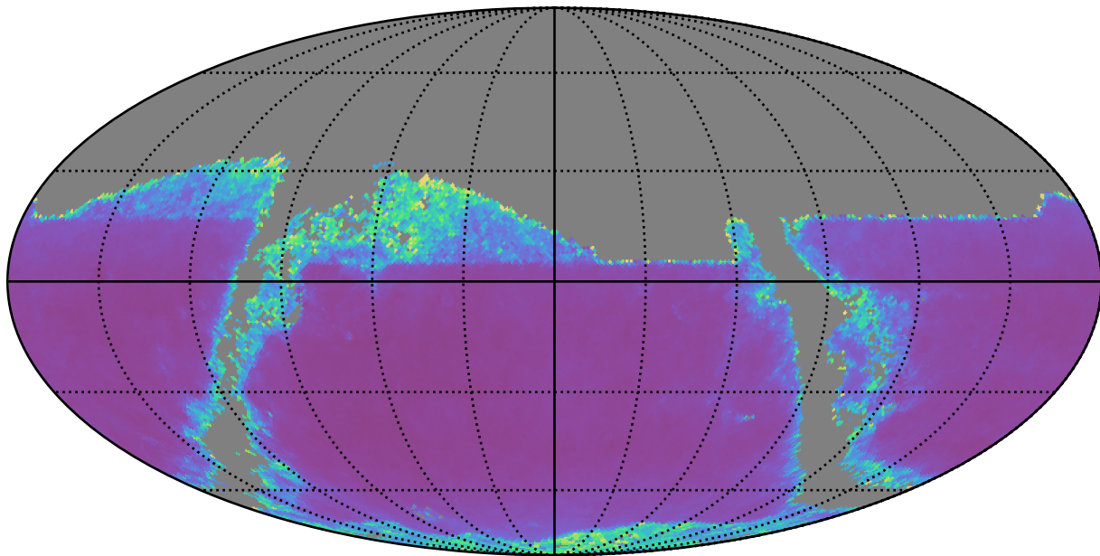
weather_cloudso16v3.4_10yrs z band: AGN SF_uncert
