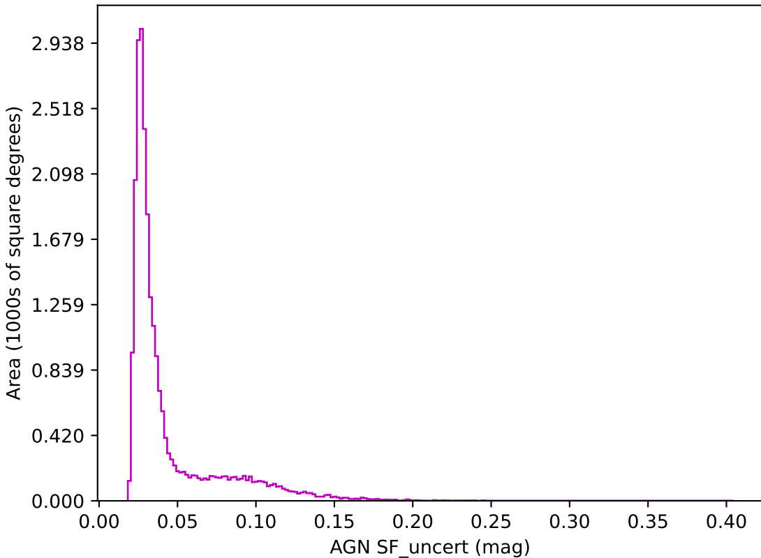
weather_cloudso16v3.4_10yrs z band: AGN SF_uncert
