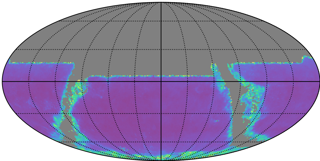
weather_cloudso16v3.4_10yrs y band: AGN SF_uncert
