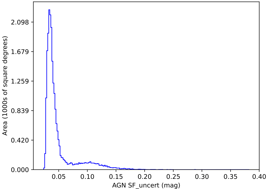
weather_cloudso16v3.4_10yrs y band: AGN SF_uncert
