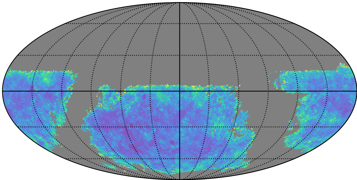
weather_cloudso16v3.4_10yrs u band: AGN SF_uncert
