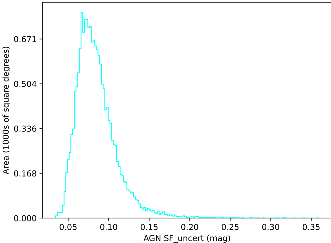
weather_cloudso16v3.4_10yrs u band: AGN SF_uncert
