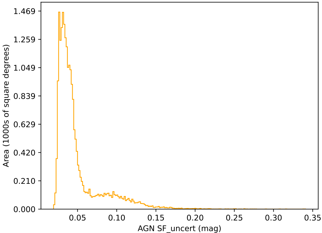
weather_cloudso16v3.4_10yrs r band: AGN SF_uncert
