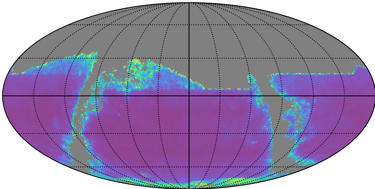
weather_cloudso16v3.4_10yrs i band: AGN SF_uncert
