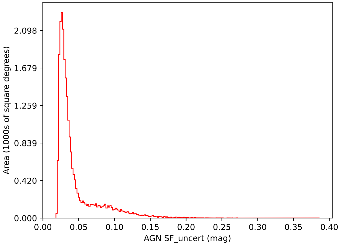
weather_cloudso16v3.4_10yrs i band: AGN SF_uncert
