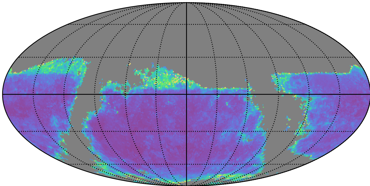
weather_cloudso16v3.4_10yrs g band: AGN SF_uncert
